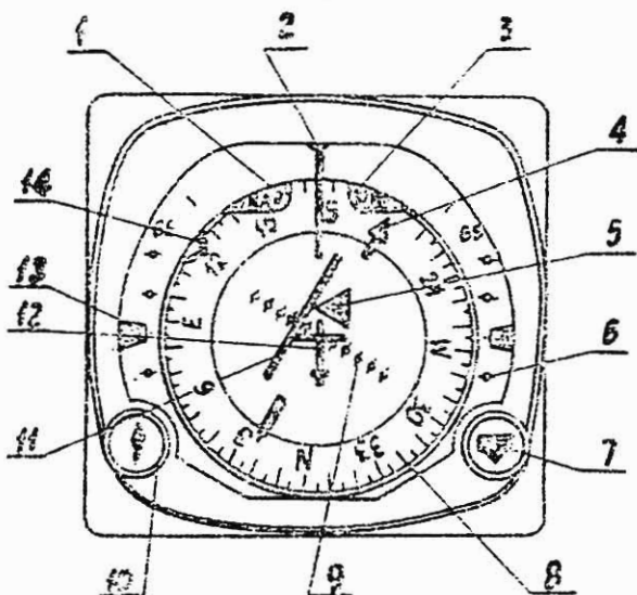
Fig. 5. YC 325A Indicator
