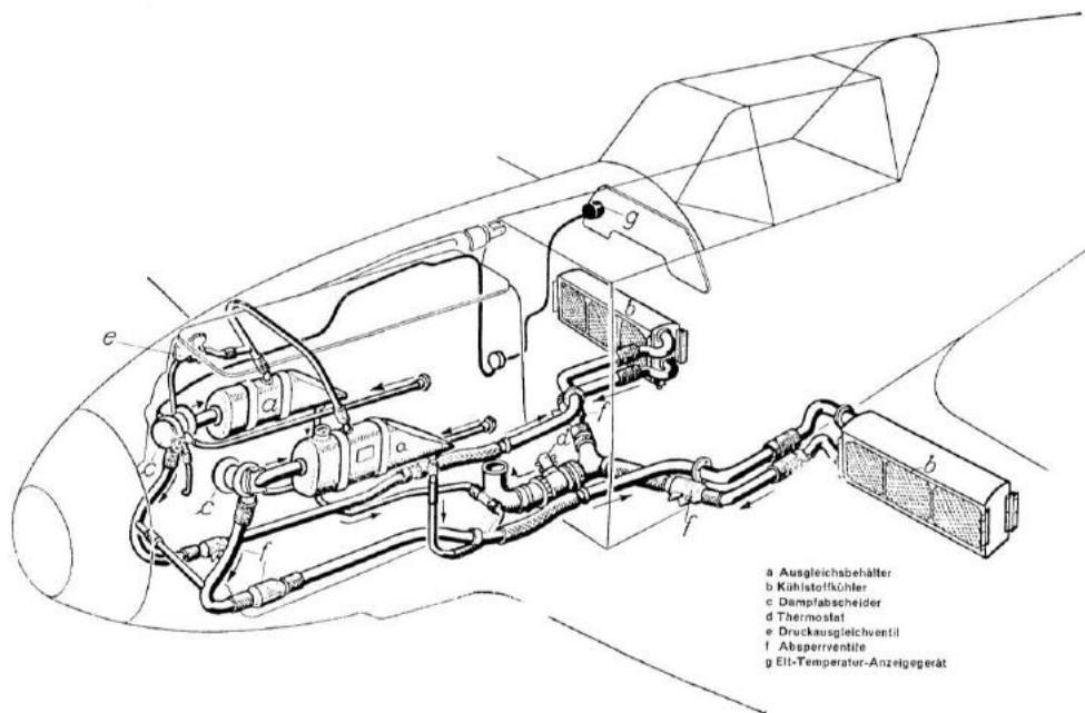
Abb. 36: Übersicht der Kühlstoffanlage
