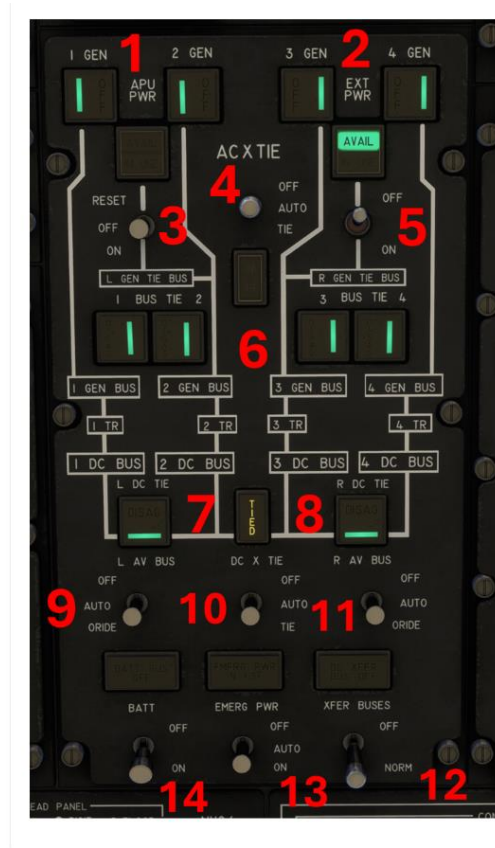
Electrical Panel (Overhead)
